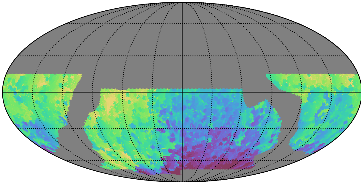
baseline_v2.0_10yrs WFD z band: Min HA
