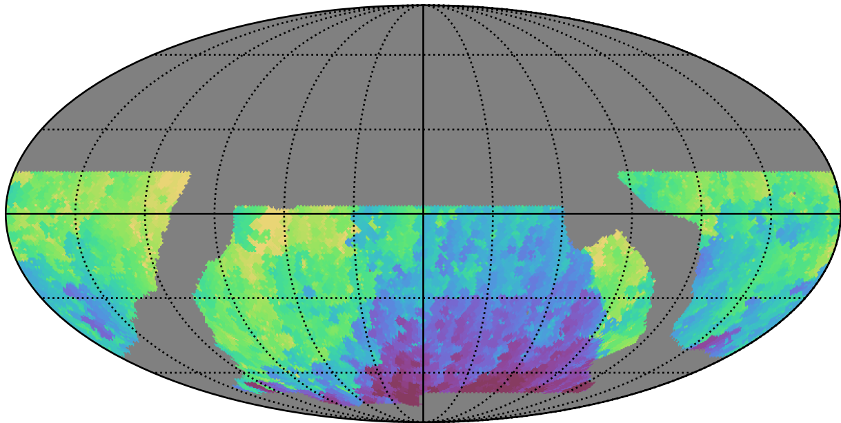
baseline_v2.0_10yrs WFD y band: Min HA
