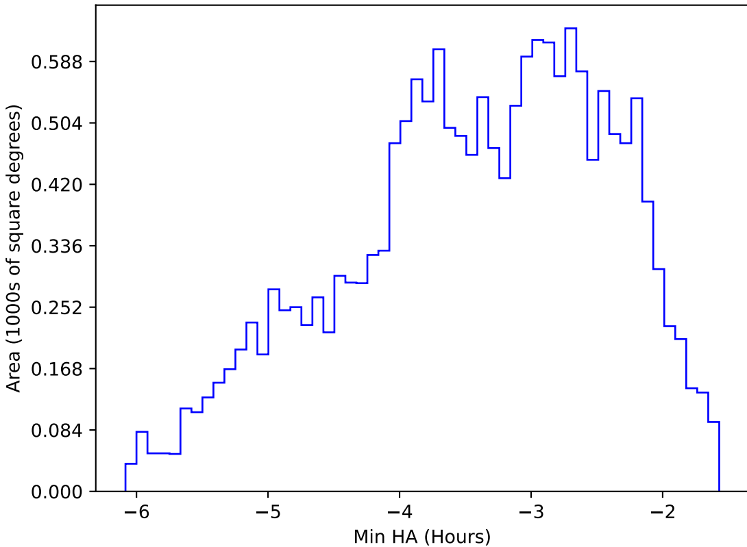
baseline_v2.0_10yrs WFD y band: Min HA
