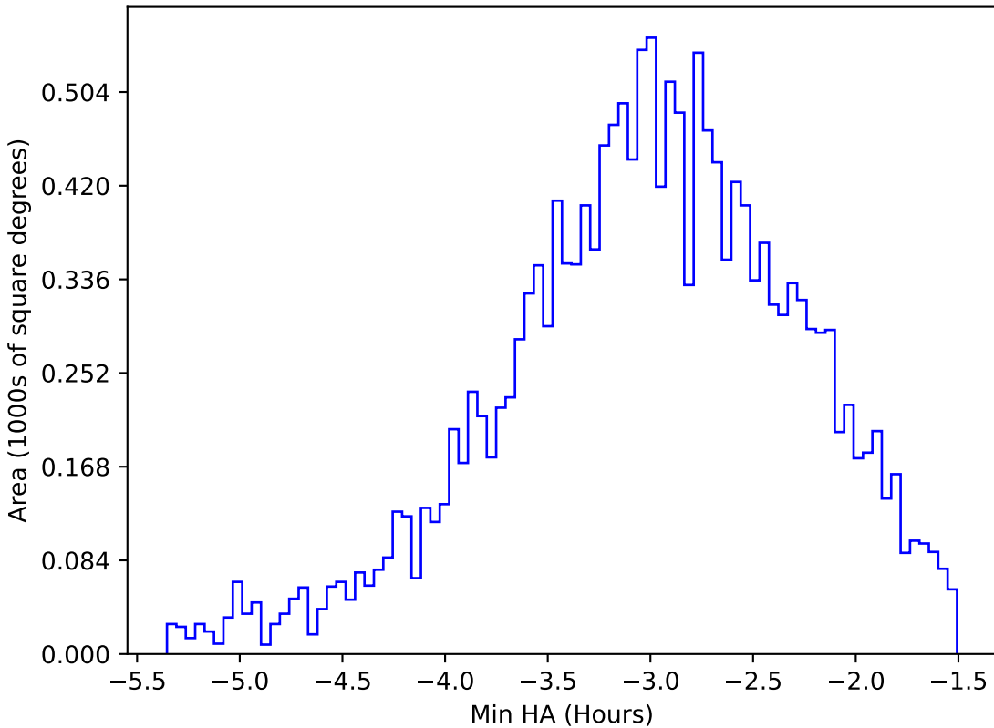
baseline_v2.0_10yrs WFD u band: Min HA
