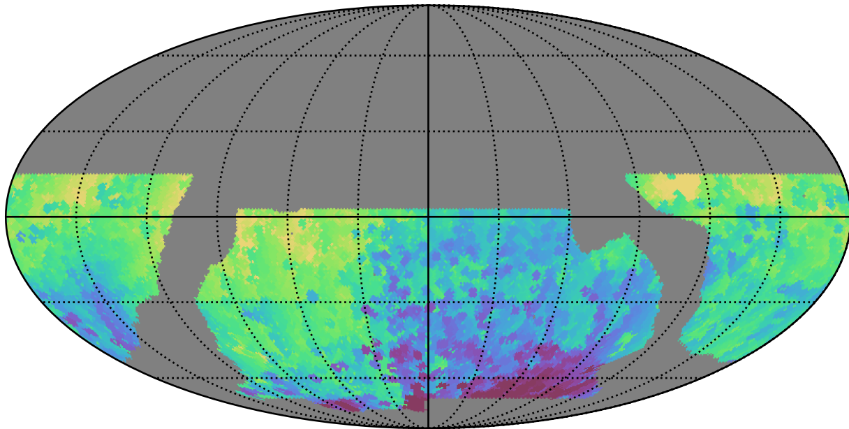
baseline_v2.0_10yrs WFD r band: Min HA
