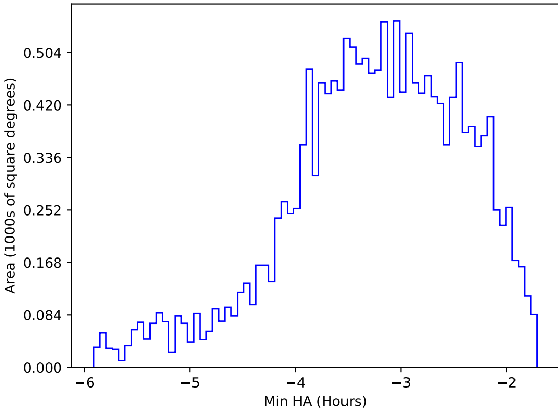
baseline_v2.0_10yrs WFD i band: Min HA
