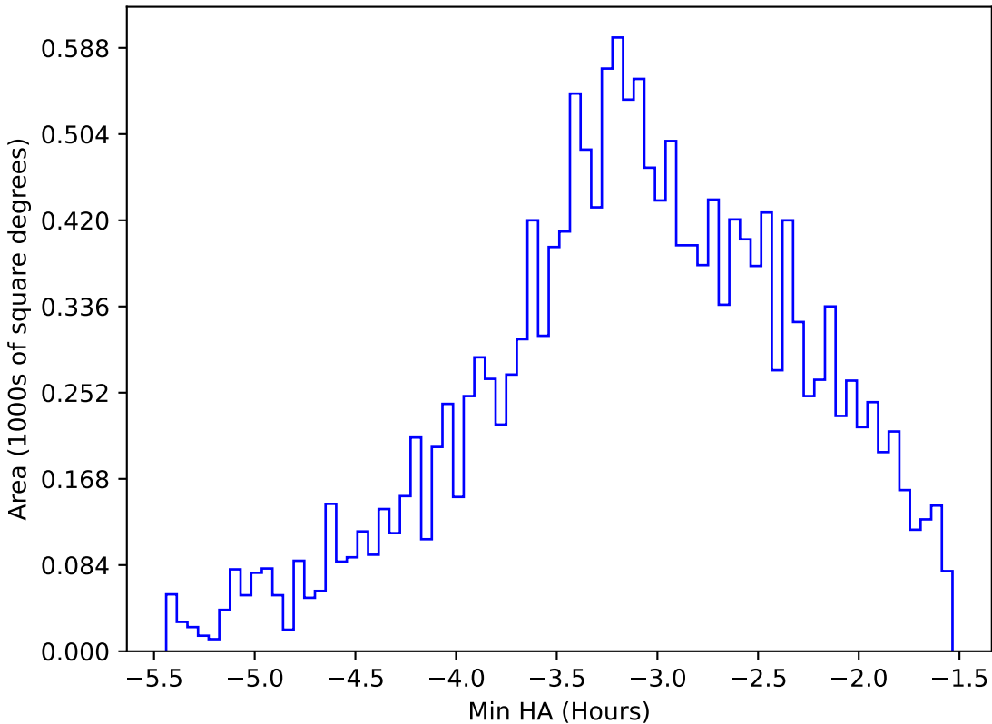
baseline_v2.0_10yrs WFD g band: Min HA
