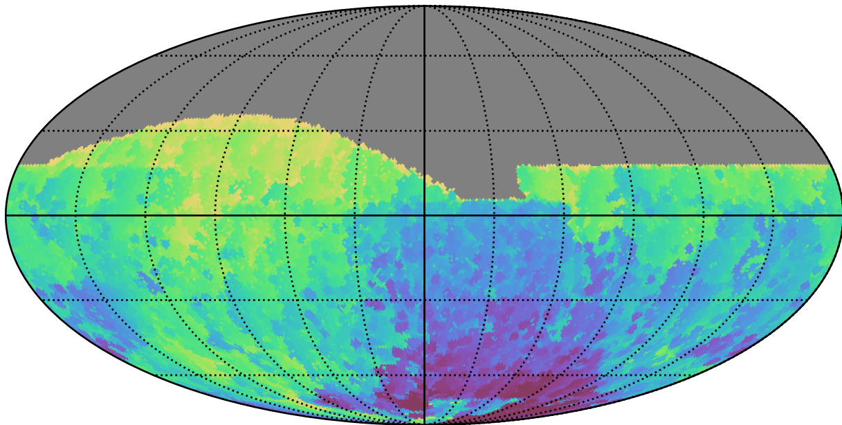
baseline_v2.0_10yrs All sky z band: Min HA
