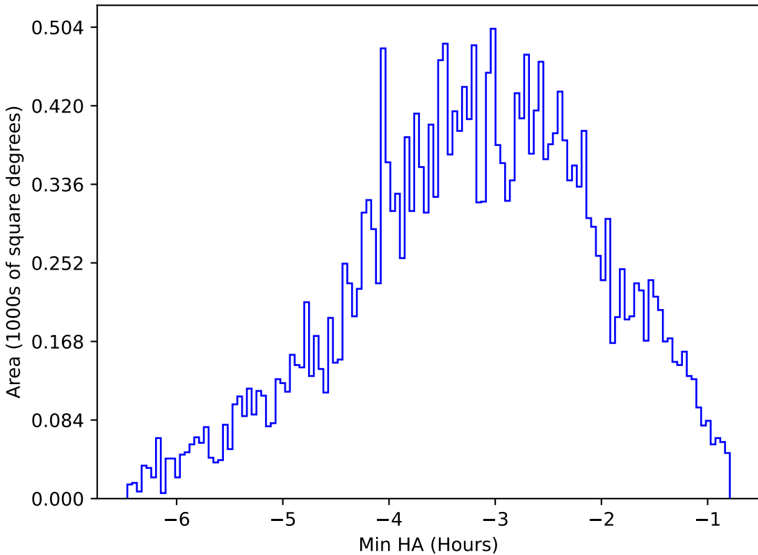
baseline_v2.0_10yrs All sky z band: Min HA
