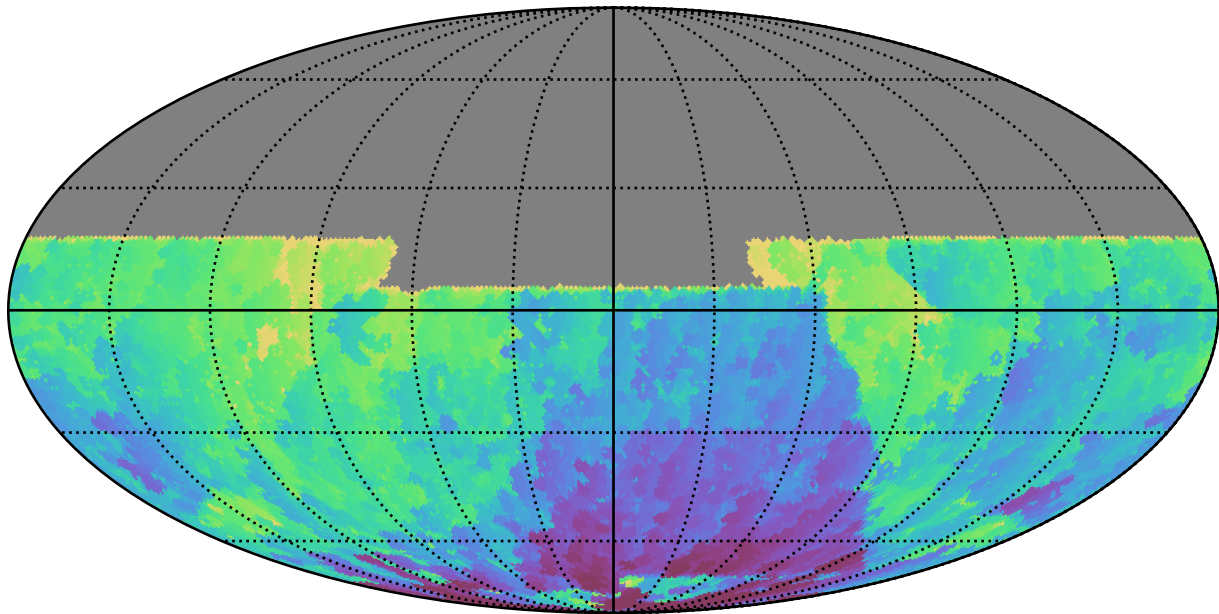
baseline_v2.0_10yrs All sky y band: Min HA
