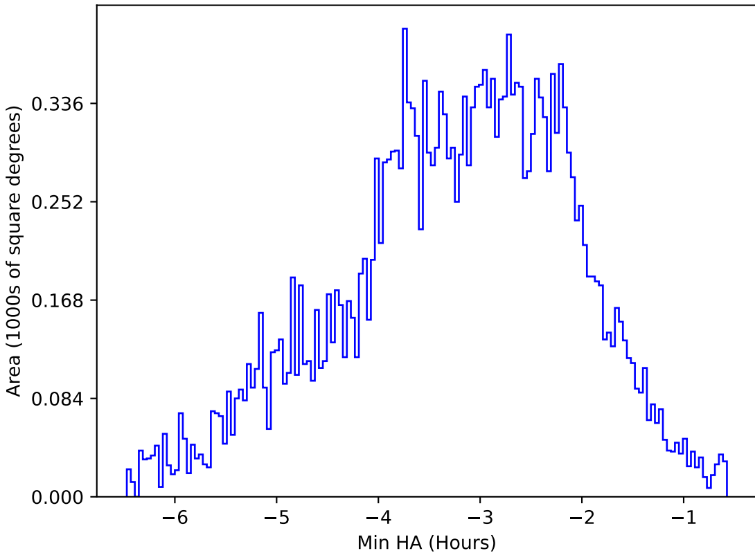
baseline_v2.0_10yrs All sky y band: Min HA
