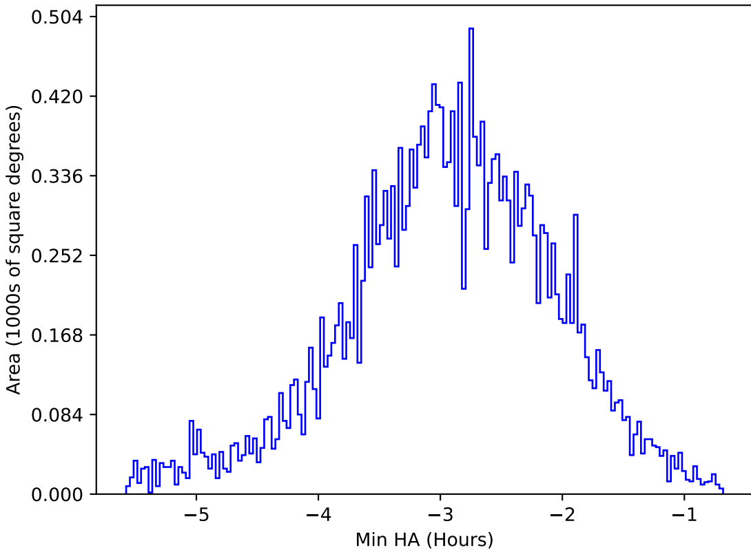
baseline_v2.0_10yrs All sky u band: Min HA
