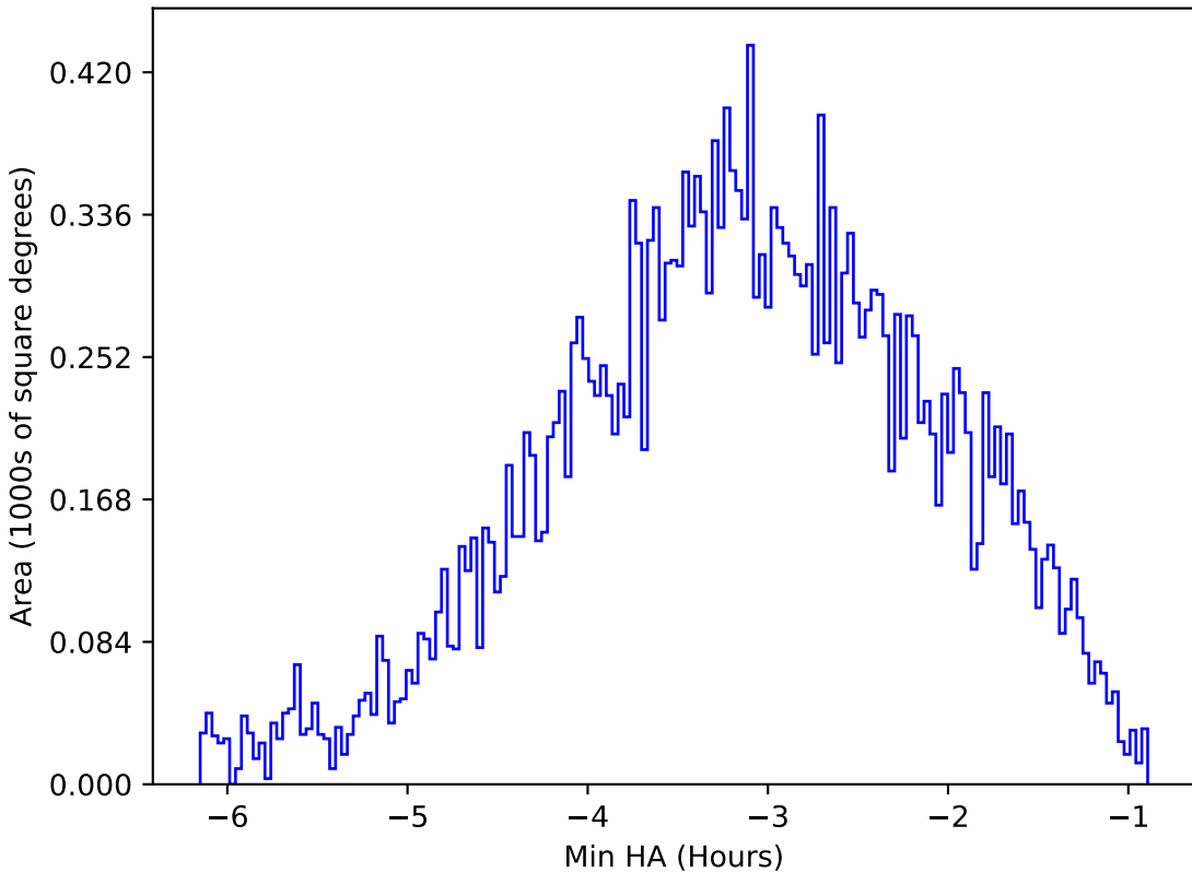
baseline_v2.0_10yrs All sky r band: Min HA
