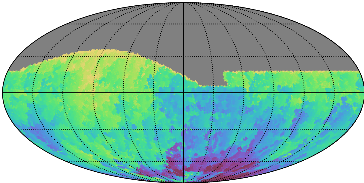
baseline_v2.0_10yrs All sky i band: Min HA
