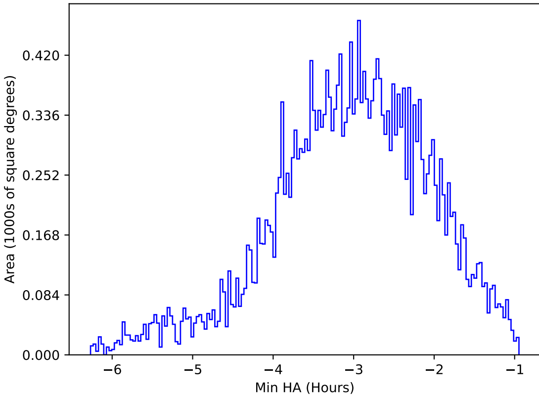
baseline_v2.0_10yrs All sky i band: Min HA
