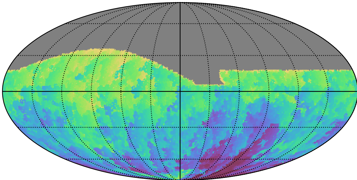
baseline_v2.0_10yrs All sky g band: Min HA
