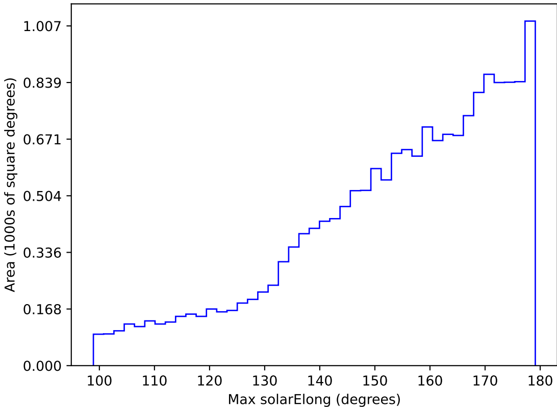
baseline_v2.0_10yrs WFD y band: Max solarElong
