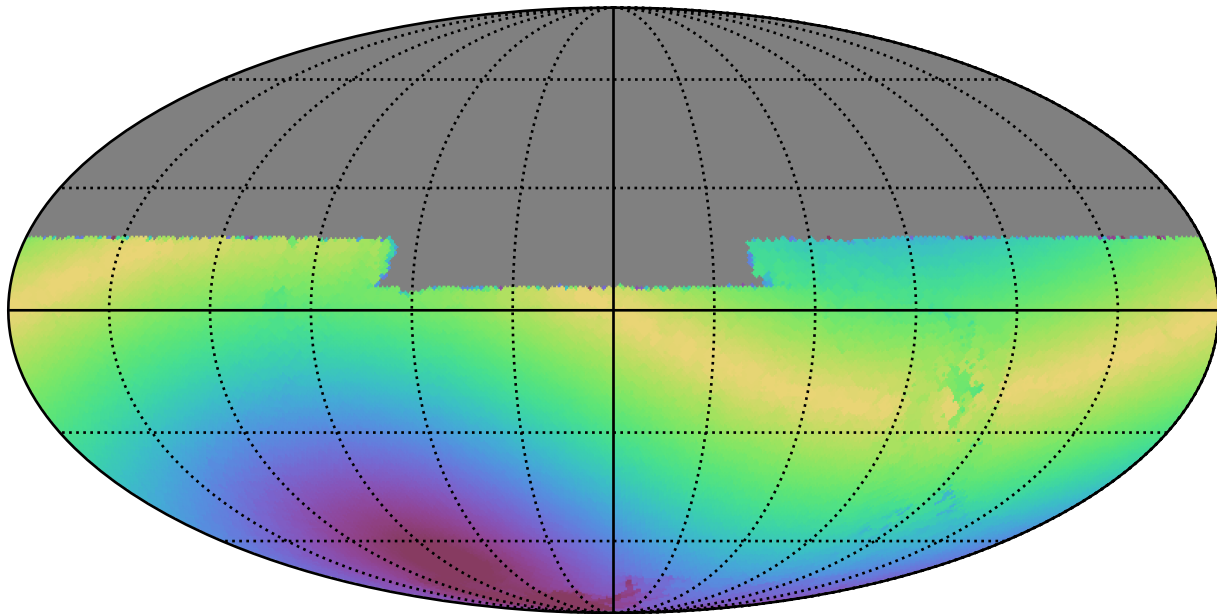
baseline_v2.0_10yrs All sky y band: Max solarElong
