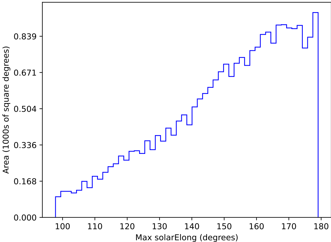
baseline_v2.0_10yrs All sky y band: Max solarElong
