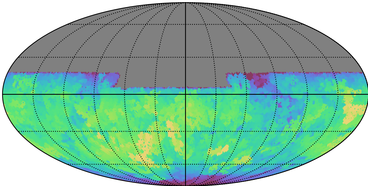
baseline_v2.0_10yrs All sky y band: Max saturation_mag
