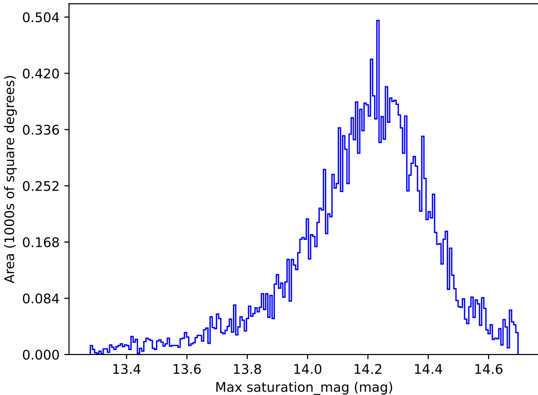
baseline_v2.0_10yrs All sky y band: Max saturation_mag
