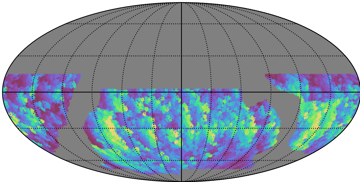
baseline_v2.0_10yrs WFD y band: Max normairmass
