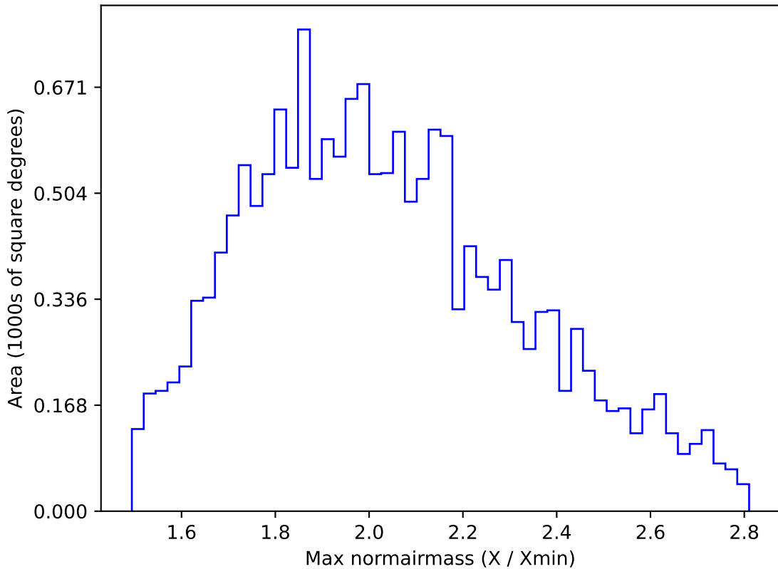
baseline_v2.0_10yrs WFD y band: Max normairmass
