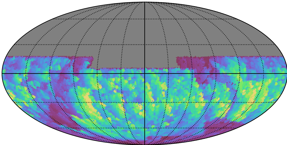
baseline_v2.0_10yrs All sky y band: Max normairmass
