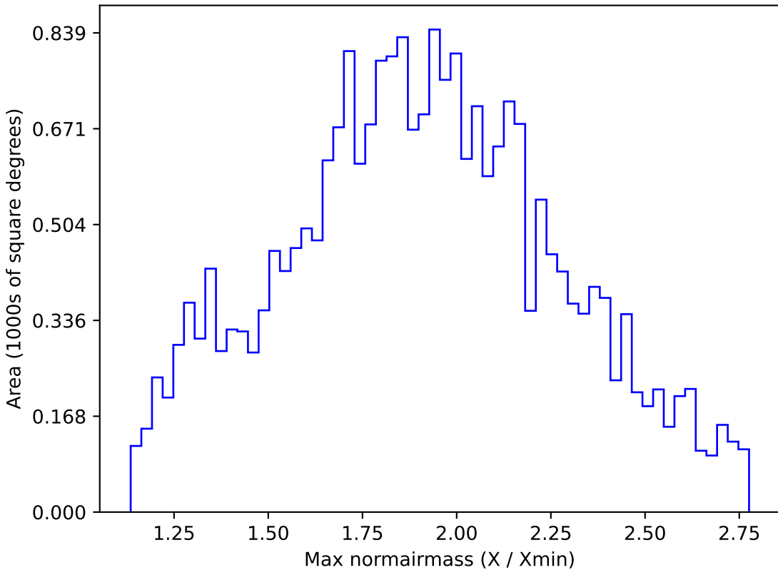
baseline_v2.0_10yrs All sky y band: Max normairmass
