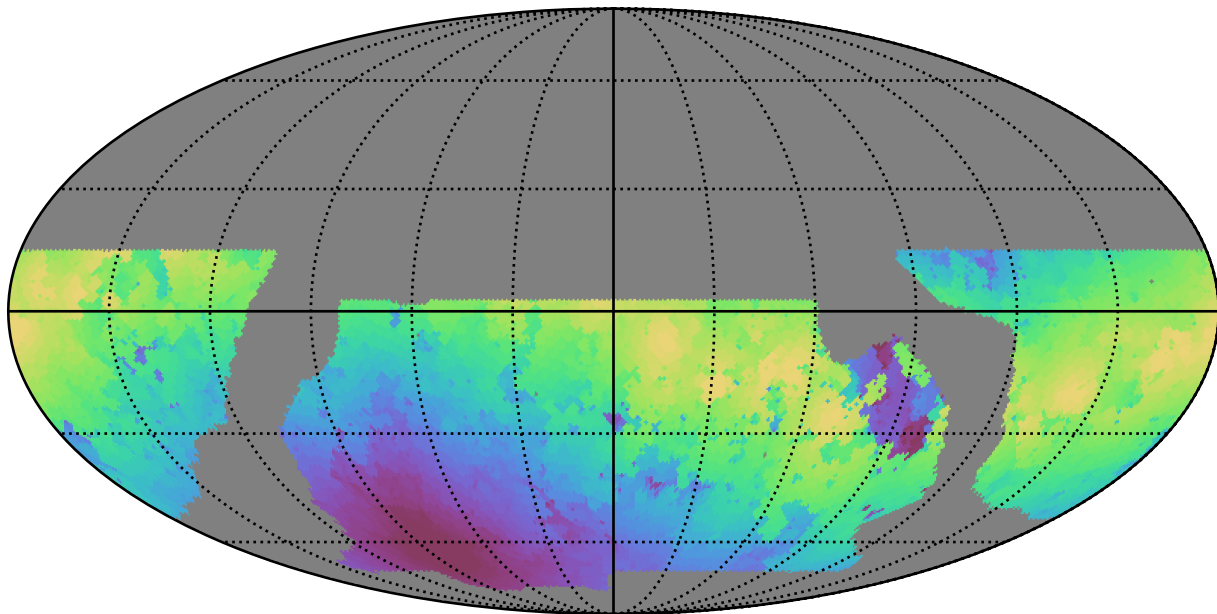
baseline_v2.0_10yrs WFD y band: Max moonDistance
