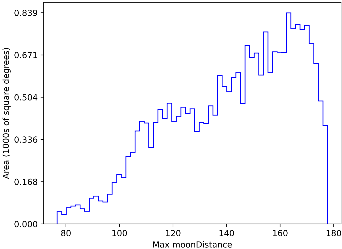
baseline_v2.0_10yrs All sky y band: Max moonDistance
