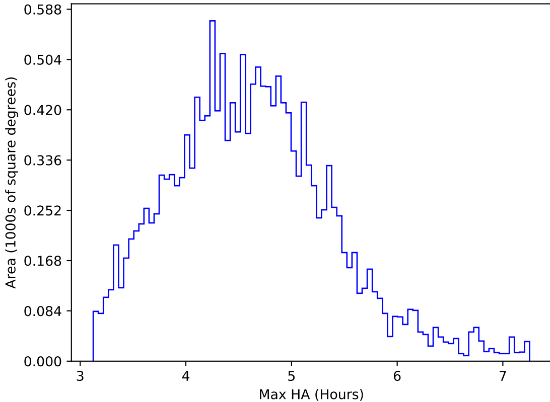
baseline_v2.0_10yrs WFD y band: Max HA
