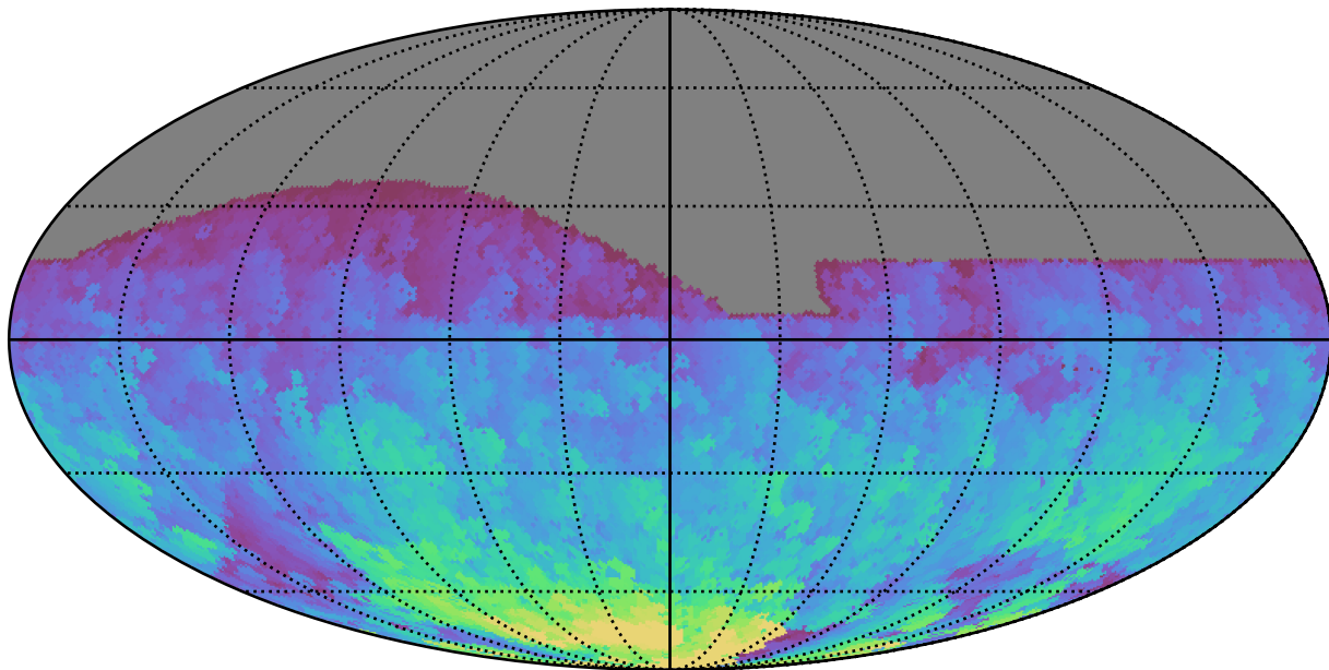
baseline_v2.0_10yrs All sky z band: Max HA
