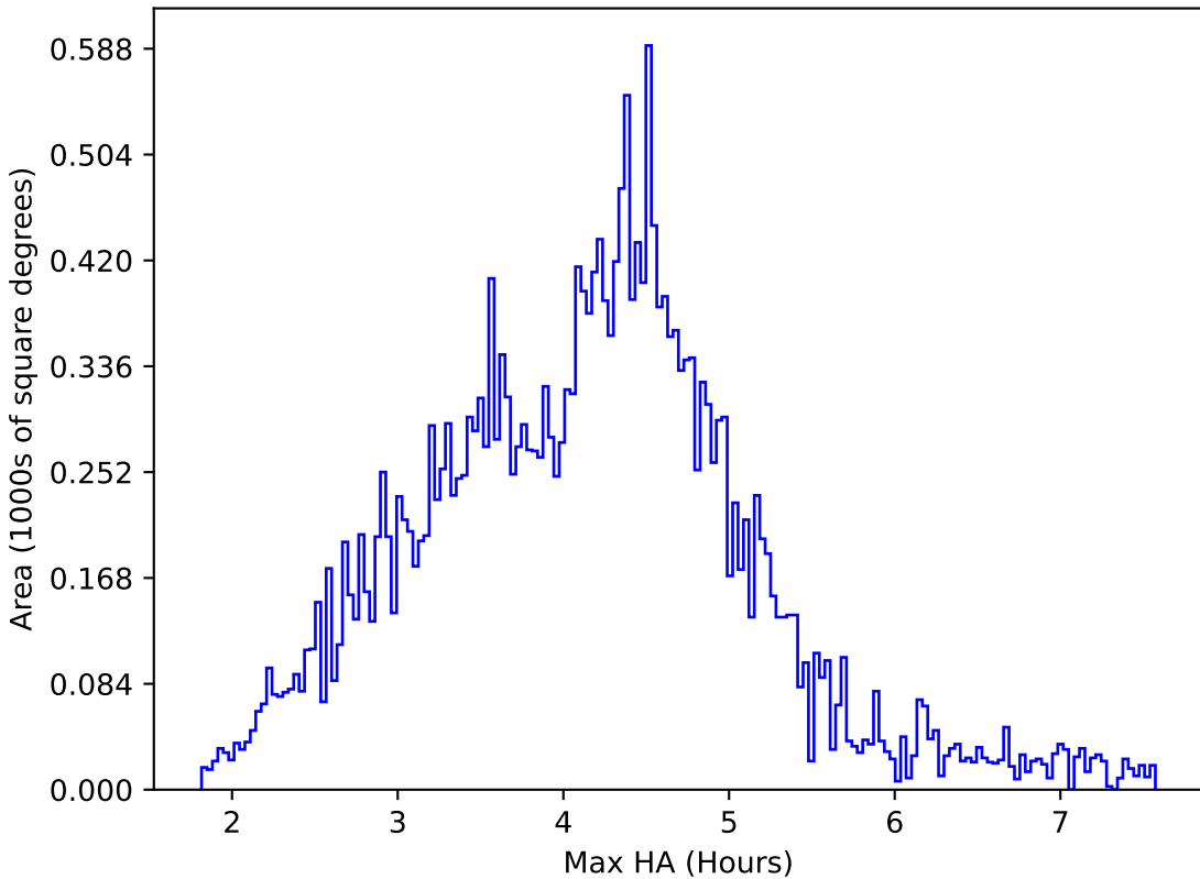
baseline_v2.0_10yrs All sky z band: Max HA
