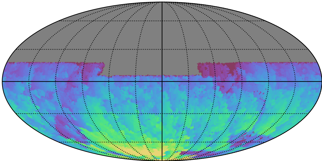
baseline_v2.0_10yrs All sky y band: Max HA
