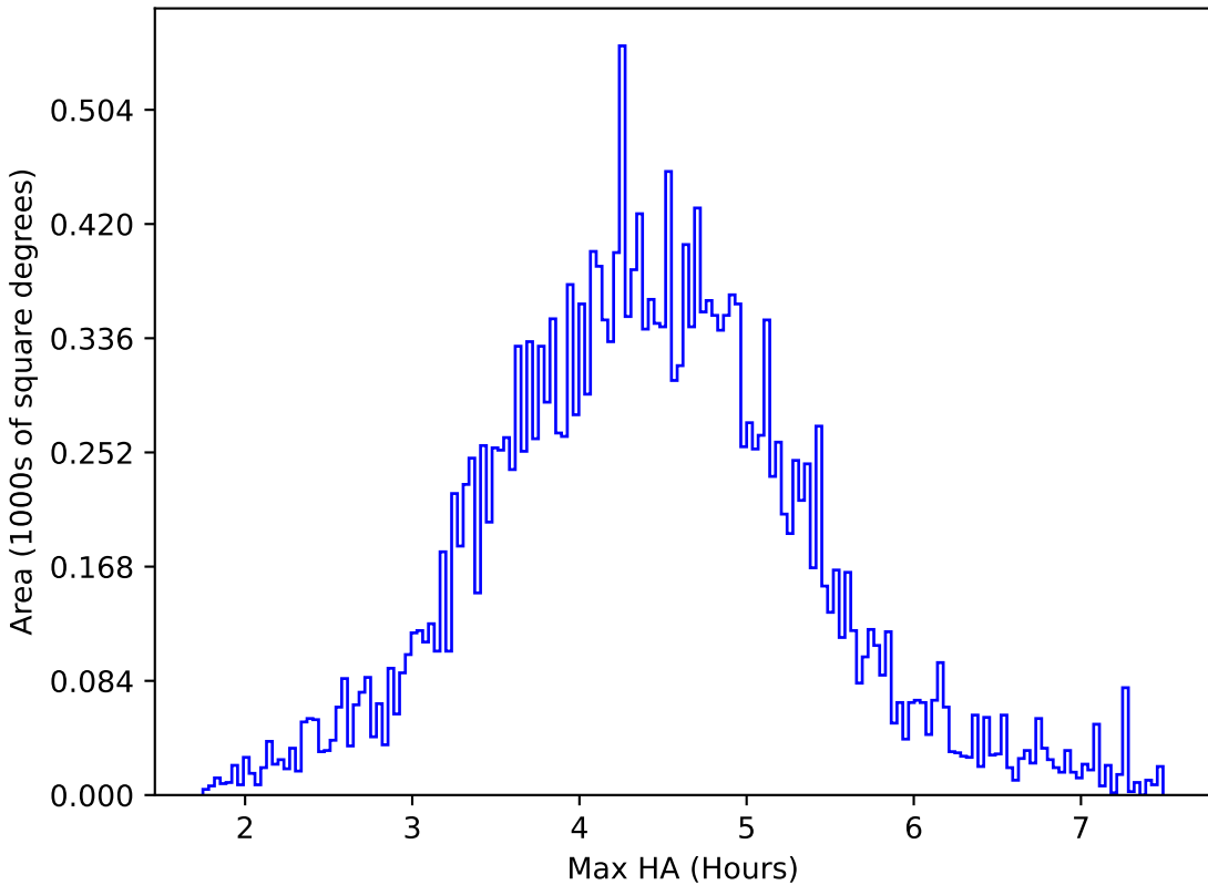
baseline_v2.0_10yrs All sky y band: Max HA
