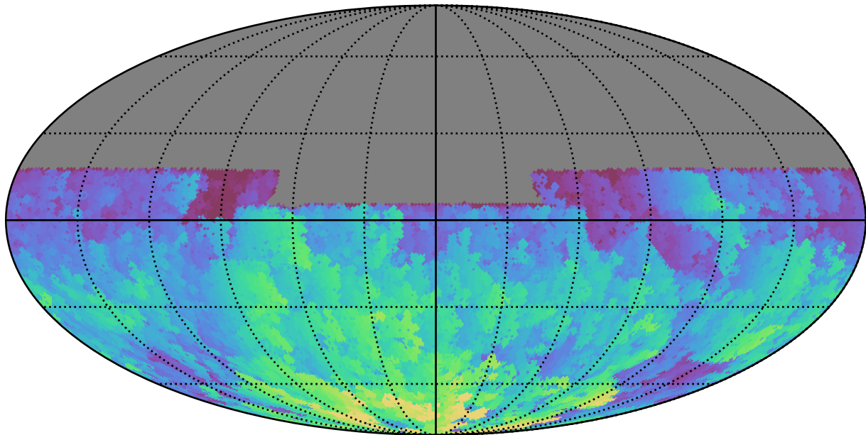
baseline_v2.0_10yrs All sky u band: Max HA
