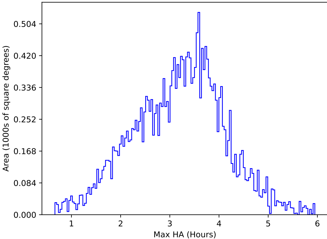
baseline_v2.0_10yrs All sky u band: Max HA
