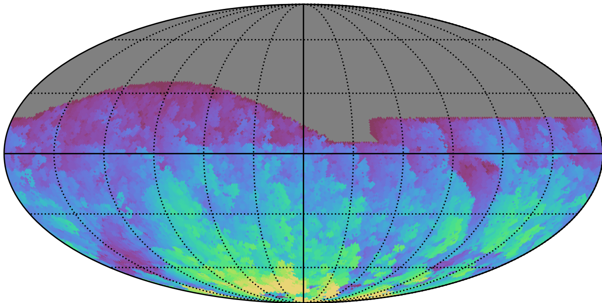
baseline_v2.0_10yrs All sky r band: Max HA
