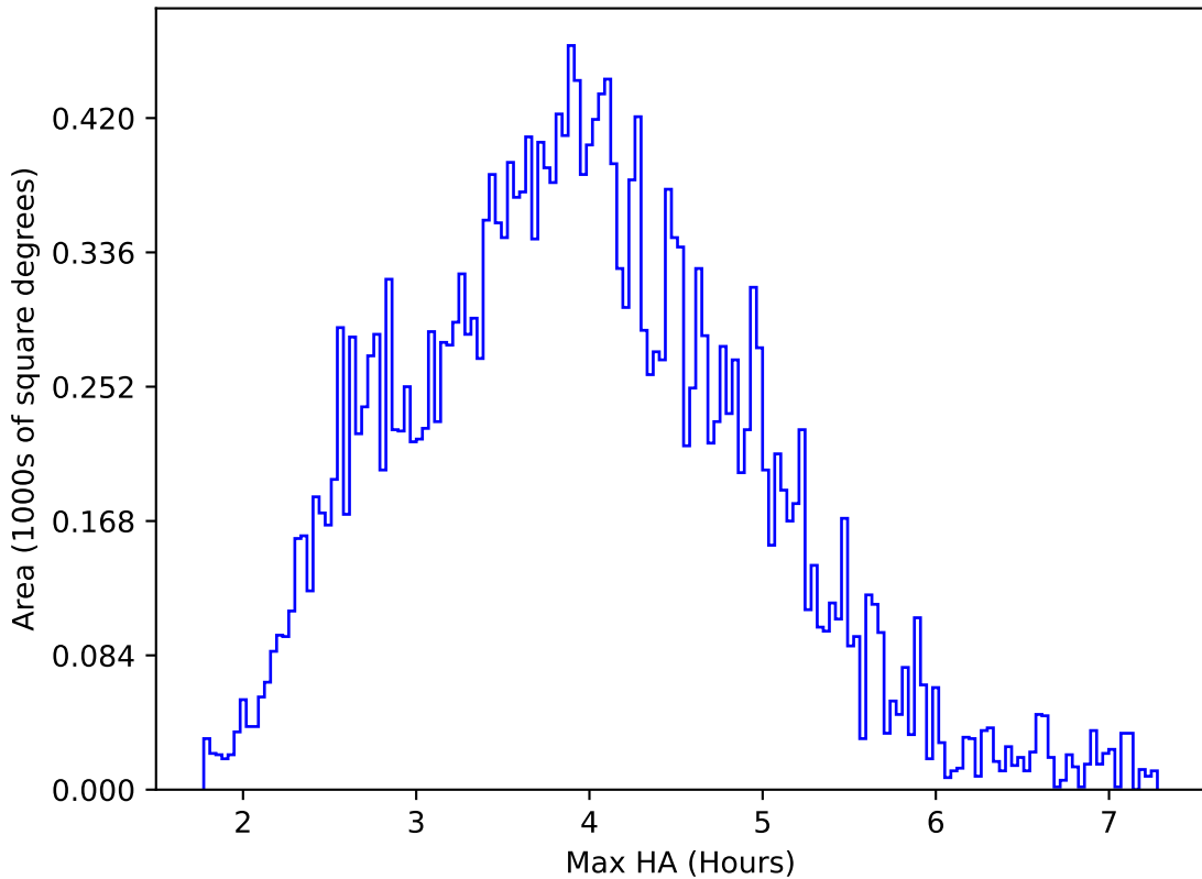
baseline_v2.0_10yrs All sky r band: Max HA
