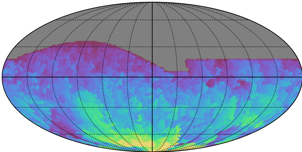
baseline_v2.0_10yrs All sky i band: Max HA
