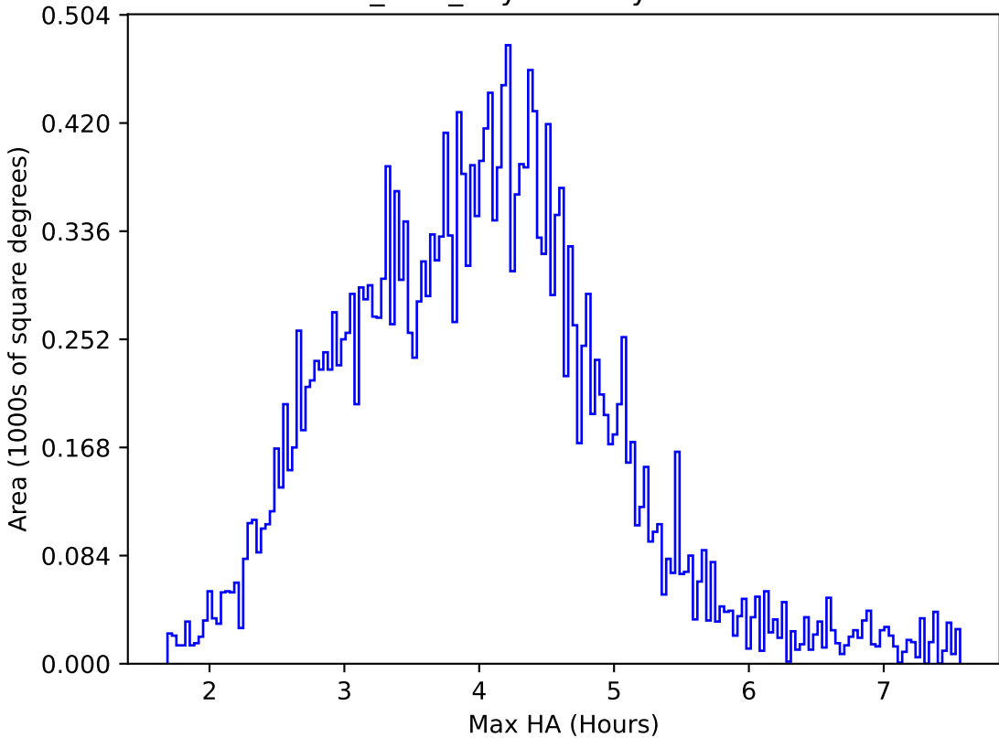
baseline_v2.0_10yrs All sky i band: Max HA
