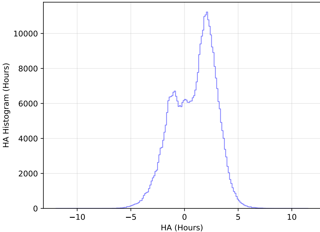
baseline_v2.0_10yrs All sky y band: HA Histogram
