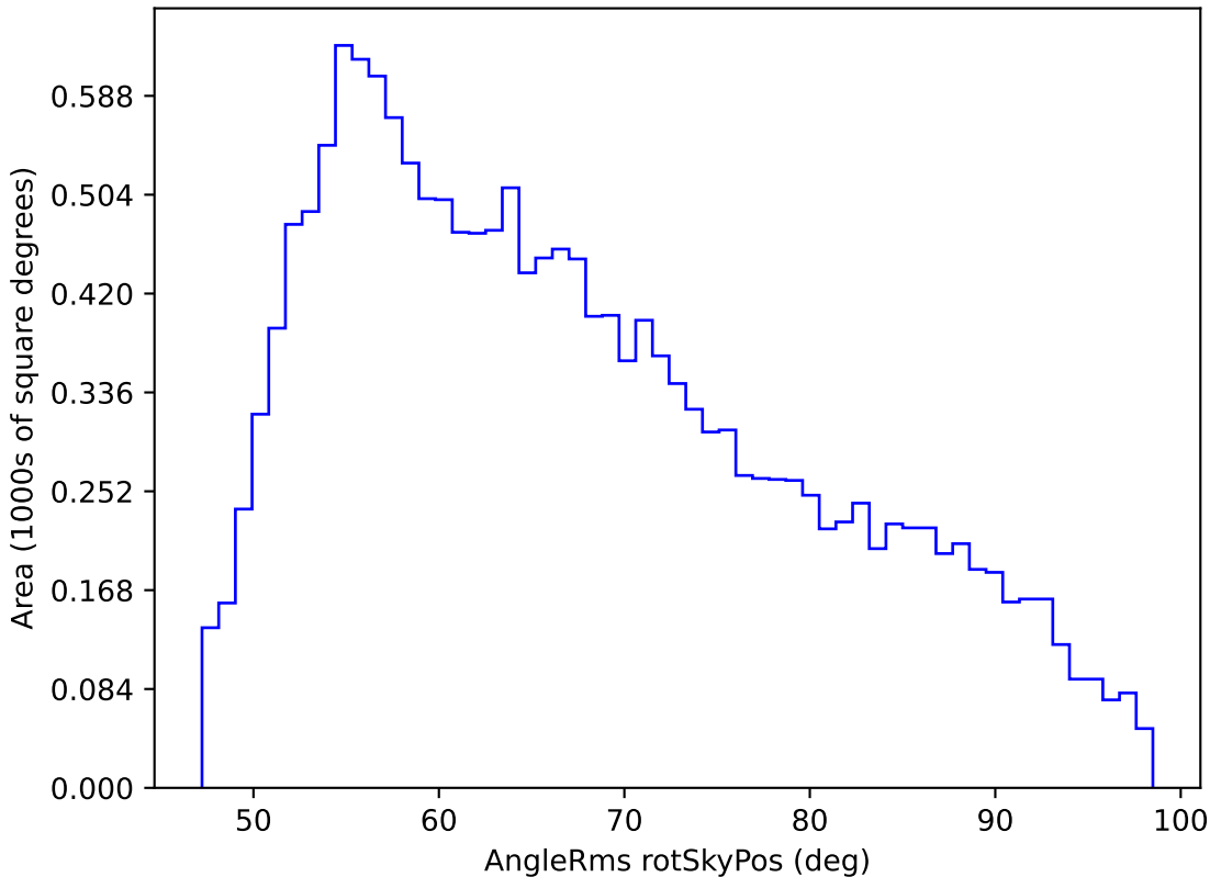
baseline_v2.0_10yrs WFD y band: AngleRms rotSkyPos
