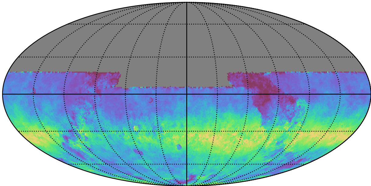
baseline_v2.0_10yrs All sky y band: AngleRms rotSkyPos
