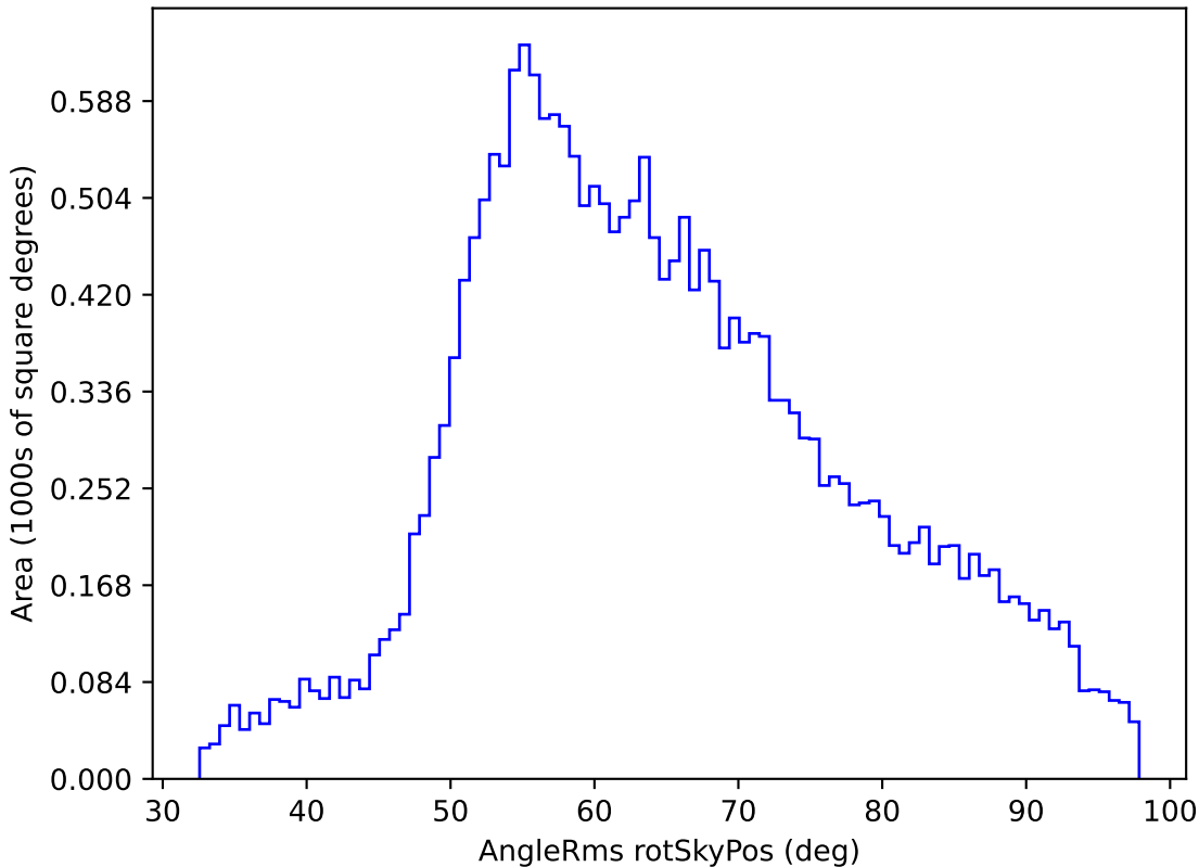
baseline_v2.0_10yrs All sky y band: AngleRms rotSkyPos
