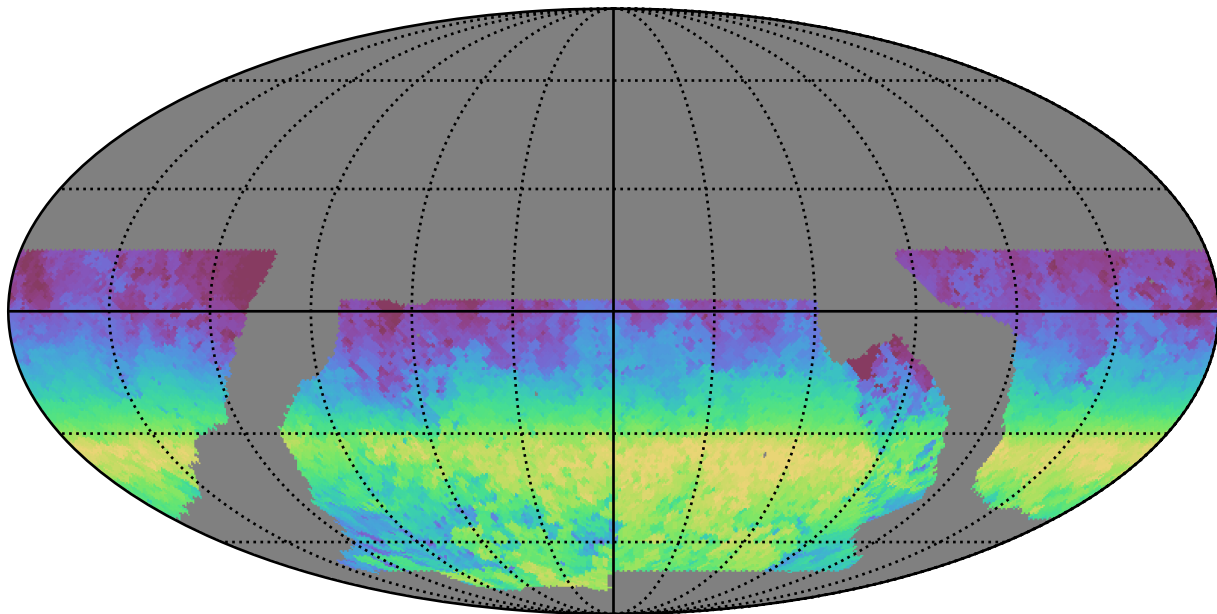
baseline_v2.0_10yrs WFD y band: AngleRange rotSkyPos
