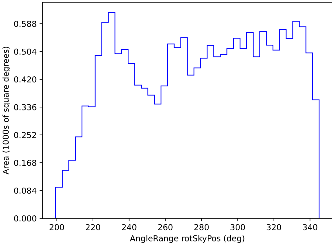
baseline_v2.0_10yrs WFD y band: AngleRange rotSkyPos
