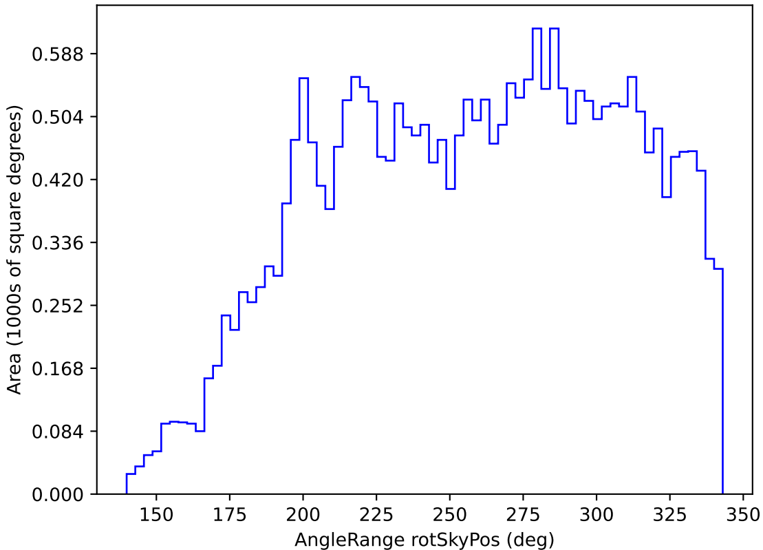
baseline_v2.0_10yrs All sky z band: AngleRange rotSkyPos
