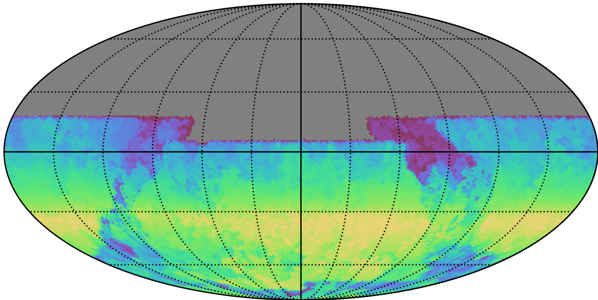
baseline_v2.0_10yrs All sky y band: AngleRange rotSkyPos
