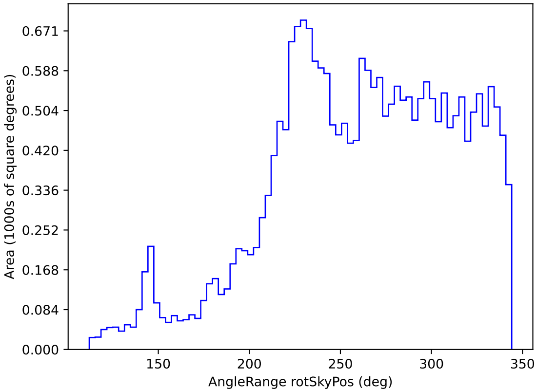
baseline_v2.0_10yrs All sky y band: AngleRange rotSkyPos
