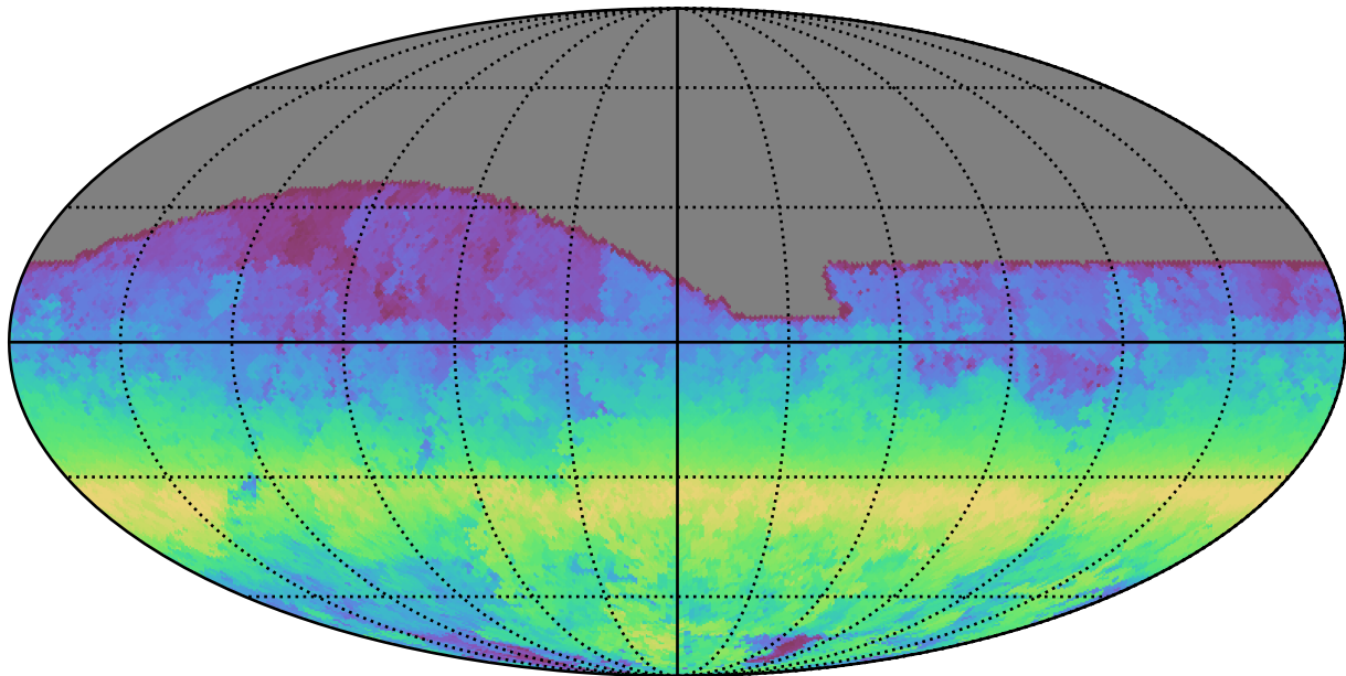
baseline_v2.0_10yrs All sky i band: AngleRange rotSkyPos
