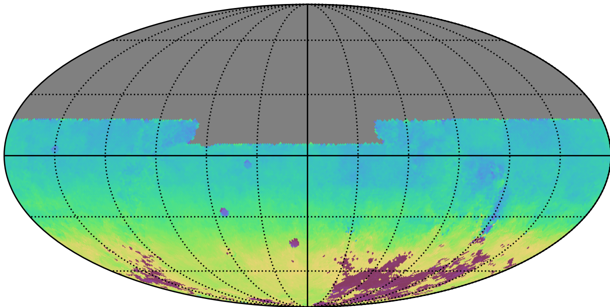
baseline_v2.0_10yrs All sky y band: AngleMean rotSkyPos
