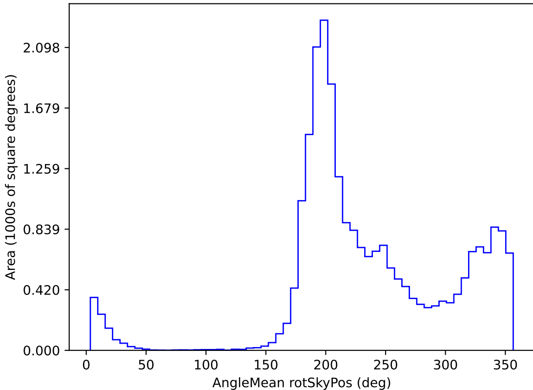
baseline_v2.0_10yrs All sky y band: AngleMean rotSkyPos
